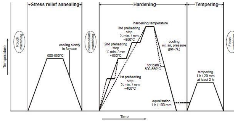
نمودار CCT
