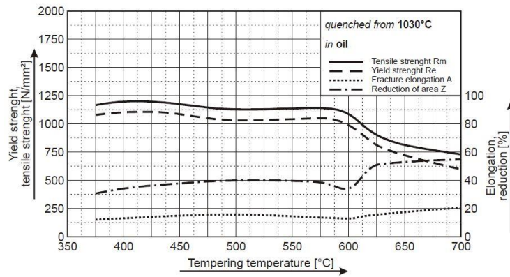
نمودار بازیخت (Temper)
