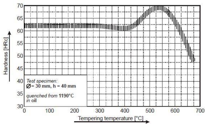
نمودار بازیخت (Temper)
